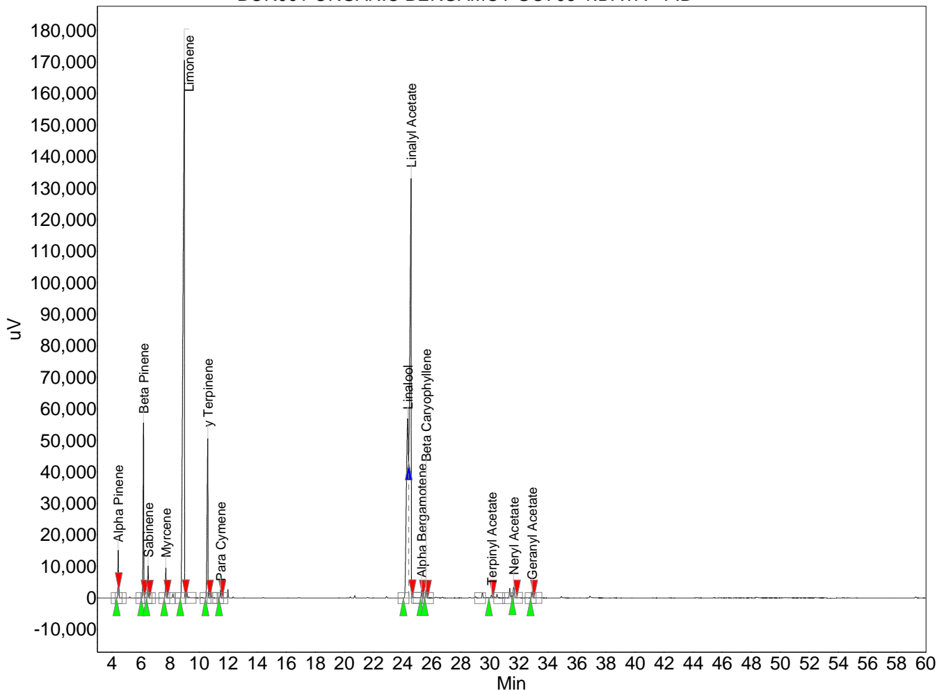
BOR001 ORGANIC BERGAMOT GO706-1.DATA - FID
